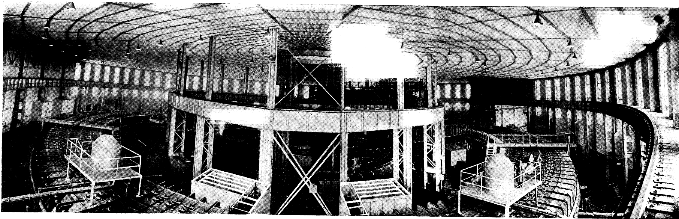
Obr. 1. Celkový pohled na sovětský synchrotrón na 10 BeV.
