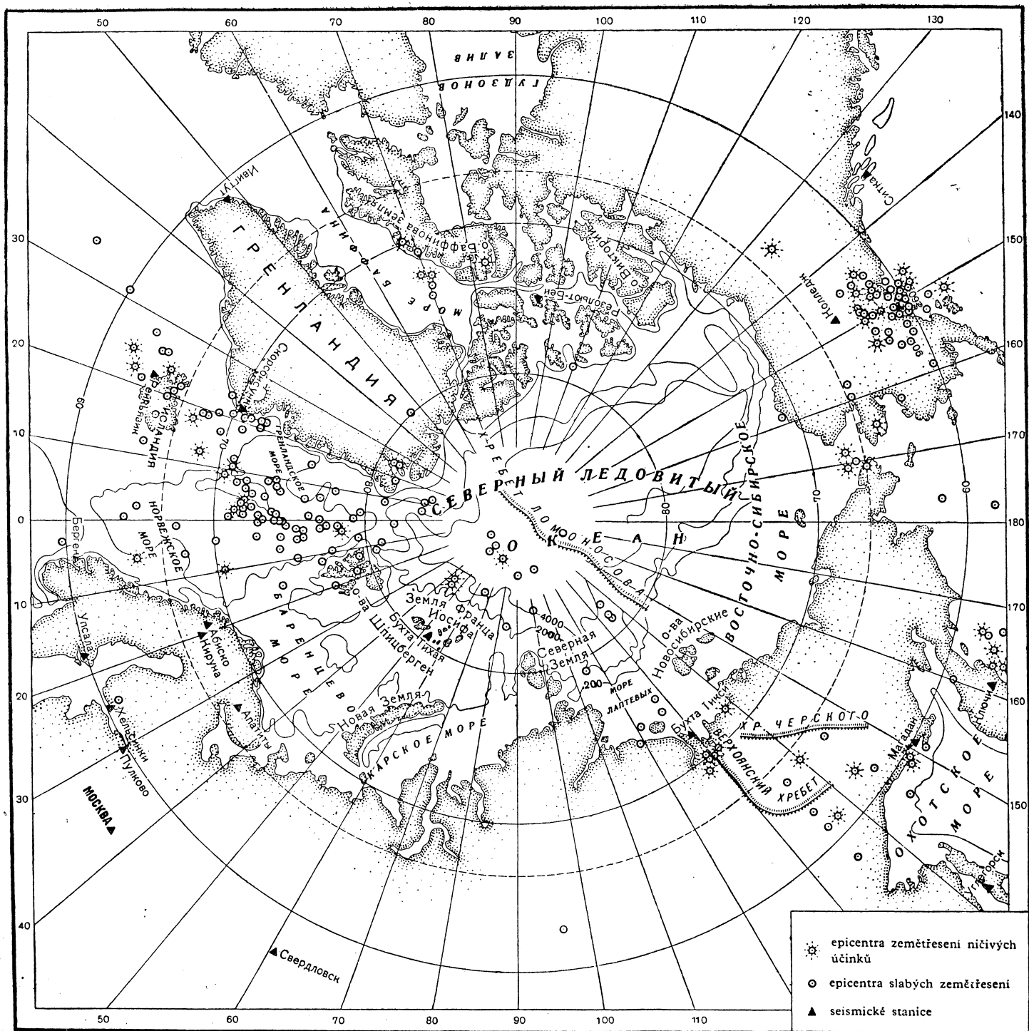
· Obr. 2. Seismicky aktivni oblast v Arktidě.
