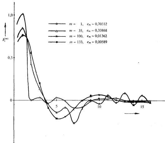
Obr. 3. Impulzné charakteristiky lineárneho modelu, \mathbf{h}_m = (h_1^{(m)}, h_2^{(m)}, \dots, h_{16}^{(m)}) , dosiahnuté pri počte iterácií m .
