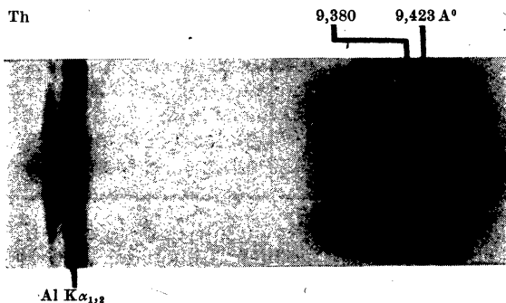
Abb. 2. Th (90): N-Serie, N_I -Untergruppe.
