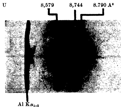
Abb. 1. U (92): N-Serie, N_I -Untergruppe.
