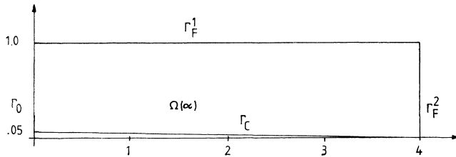
Fig. 7.8. \Omega(\alpha) , \alpha \in \mathcal{Q}_{\text{ad}}^1 .
