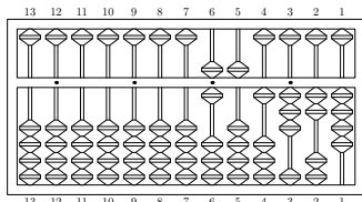
(a) Nastavíme 651 324.
