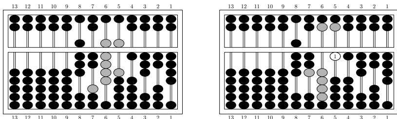
Obrázek 5: Zvýraznění všech přesunů v jednom z mezikroků při sčítání 829\,513\,24 + 60\,000 . Všechny korálky, které byly přesunuty, jsou vykresleny šedou barvou, a navíc jsme si vyznačili aktuální hodnotu na tyčce, se kterou bylo pracováno. V našem případě to byla hodnota 60\,000 , tedy pátá tyčka.
