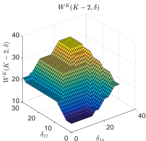
Fig. 7. W^K(K, \delta) .
