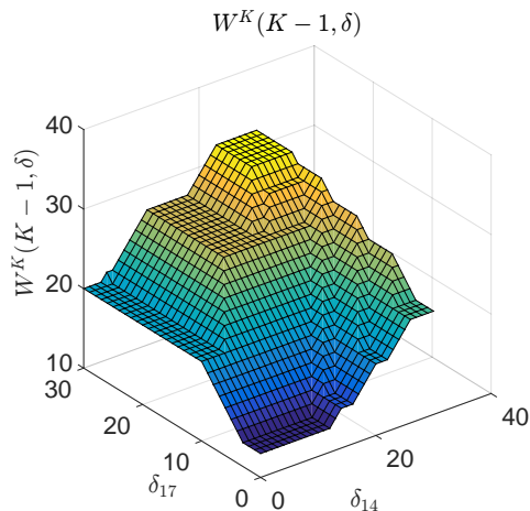
Fig. 6. W^K(K-1, \delta) .
