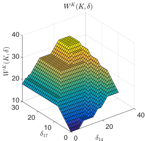
Fig. 5. W^K(K, \delta) .
