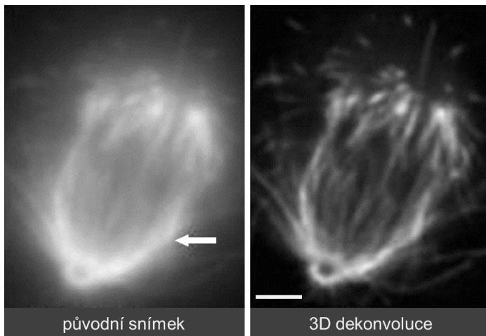
Obr. 3. Ukázka použití 3D dekonvoluce k potlačení neostrých obrazů z mimoohniskových rovin: dělicí se žabí buňka z tkáňové kultury XLK2 odvozené od larválních ledvin (fluorescenční mikroskopie imunofluorescenčně označených mikrotubulů mitotického vřeténka). K dekonvoluci byla použita data z celkem 70 obrázků buňky snímaných s vertikálním krokem 0.2 \mu\text{m} . Původní snímek vlevo představuje náhodně vybraný optický řez blízko středu buňky, vpravo je obraz jemu odpovídající zaostřené roviny, který byl pomocí 3D dekonvoluce zbavený pozadí pocházejícího od neostrých obrazů sousedních rovin. Velikost bílé úsečky je 2 \mu\text{m} . Bílá šipka se týká dalších obrázků z původní publikace, zde nevyužitých. Upraveno podle [41].
