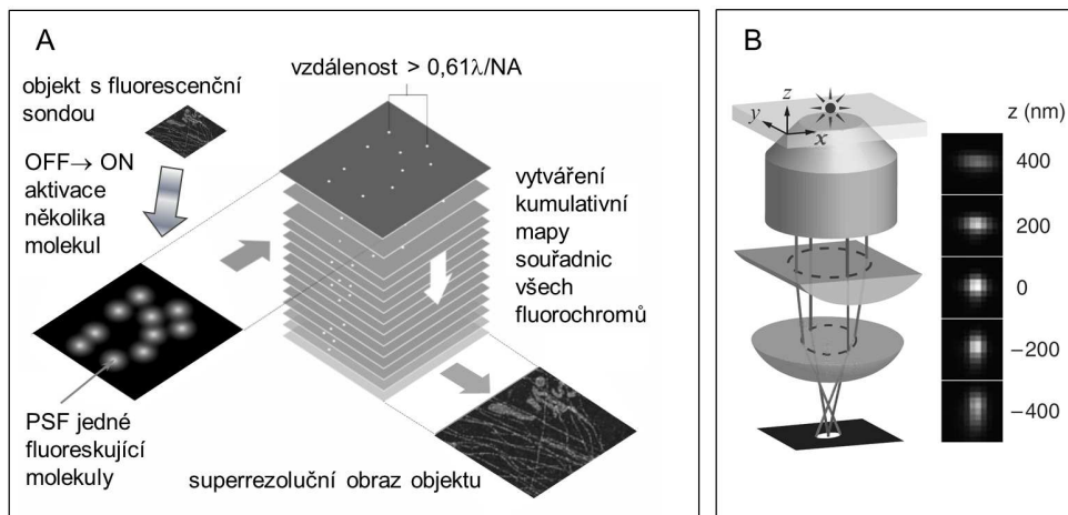
Obr. 7. Princip lokalizační superrezoluční mikroskopie. A. V objektu obsahujícím fotoaktivovatelnou nebo fotoregulovatelnou fluorescenční sondou je malý počet nahodile vybraných a dostatečně navzájem vzdálených fluorochromů přepnut aktivacím světelným pulzem do fluorescenčního stavu. Z jejich centroidních souřadnic je pak po několika desítkách tisíc opakování takové lokalizace vytvořen superrezoluční obraz distribuce fluorescenční sondy ve studovaném objektu. B. Axiální lokalizace fluorochromů použitá ve 3D STORM. Zjednodušené optické schéma ilustruje princip určení z-souřadnice fluorochromu z astigmatické formy PSF vznikající po vložení válcové čočky před projekční čočku promítající PSF na citlivou EMCCD kameru (electronmultiplying charge-coupled device). Vpravo je vertikální kalibrace elipticity astigmatické PSF. Upraveno podle [22].
