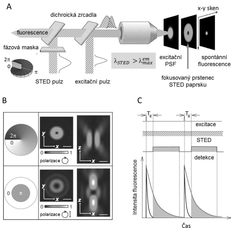
Obr. 9. Princip STED mikroskopie. A. Pulzní STED mikroskopie používající dva kolinéární laserové paprsky synchronizovaných pulzních laserů (excitační paprsek a redukční STED paprsek), které jsou fokusovány stejným objektivem na skenovaný vzorek. STED pulz vyvolávající stimulovanou emisi následuje bezprostředně po pulzu excitačním a jeho ohniskový profil (definovaný průchodem paprsku přes fázovou masku) má podobu prstence. Na panelech napravo od objektivu jsou schematicky znázorněny profily intenzit excitačního paprsku, STED paprsku a redukované spontánní fluorescence. V periferní zóně excitované oblasti vzorku byly fluorochromy deexcitovány stimulovanou emisí vyvolanou prstencovým STED paprskem. B. Vztah mezi tvarem fázové masky a 3D distribucí intenzity v ohnisku redukujícího STED paprsku. Nahoře je spirální maska umožňující dosáhnout velkého laterálního rozlišení, avšak bez vertikální selekce ve směru osy z . Dole je maska anulární, která naopak umožňuje redukcí excitovaných fluorochromů ve vertikálním směru, ovšem za cenu horšího laterálního rozlišení. Barevná verze obrázku je k dispozici pouze v online verzi tohoto článku. Upraveno podle [14]. C. Časová posloupnost excitace a detekce při hradlované STED mikroskopii. Excitace má podobu pulzů o šířce výrazně menší, než je střední doba dohasínání spontánní fluorescence, a STED paprsek má konstantní intenzitu, která se v čase nemění. Fluorescence je registrována se zpožděním T_g za excitačním pulzem, když intenzita rychleji dohasínající fluorescence fluorochromů ozařovaných STED paprskem se již blíží k nule (černá křivka), zatímco spontánní fluorescence z centra excitační stopy, kde nedochází ke stimulované emisí, má ještě stále dostatečně vysokou intenzitu (šedá křivka s výplní).
