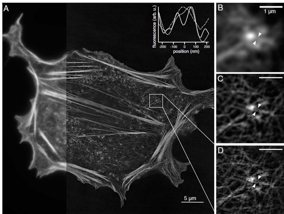
Obr. 6. Aktinový cytoskelet savčí CHO buňky (jedná se o buněčnou linii odvozenou z křeččích vaječníků) označený fotokonverzním fluorescenčním proteinem Dronpa a zobrazený nelineární NL-SIM metodou s použitím TIRF mikroskopu (Total Internal Reflection Fluorescence: fluorescence vzorku je excitována evanescentní vlnou v submikronové vrstvě přiléhající ke krycímu sklíčku). A. Celoplošný NL-SIM obraz vzorku; vlevo je ukázka kvality zobrazení pomocí obyčejné TIRF mikroskopie. Následují zvětšené obrázky čtvercové výšece porovnání B. obyčejnou celoplošnou TIRF mikroskopií, C. lineární SIM metodou a D. nelineární NL-SIM metodou. Graf normalizovaných profilů jasu mezi šipkami obrázků B–D vložený do A ukazuje, že dvě vlákna nacházející se mezi těmito šipkami jsou zřetelně rozlišena pouze v případě NL-SIM metody (plná linie), zatímco v případě obyčejné TIRF metody (tečkovaná linie) ani lineární SIM metody (čárkovaná linie) je rozlišit nejde. Převzato z [32].
