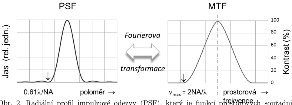
Obr. 2. Radiální profil impulzové odezvy (PSF), který je funkcí prostorových souřadnic, a modul jeho Fourierovy transformace (neboli MTF), který je funkcí prostorových frekvencí. Čárkovaná úsečka indikuje hodnotu MTF, která odpovídá prostorové frekvenci rovnající se převrácené hodnotě průměru Airyho disku.
