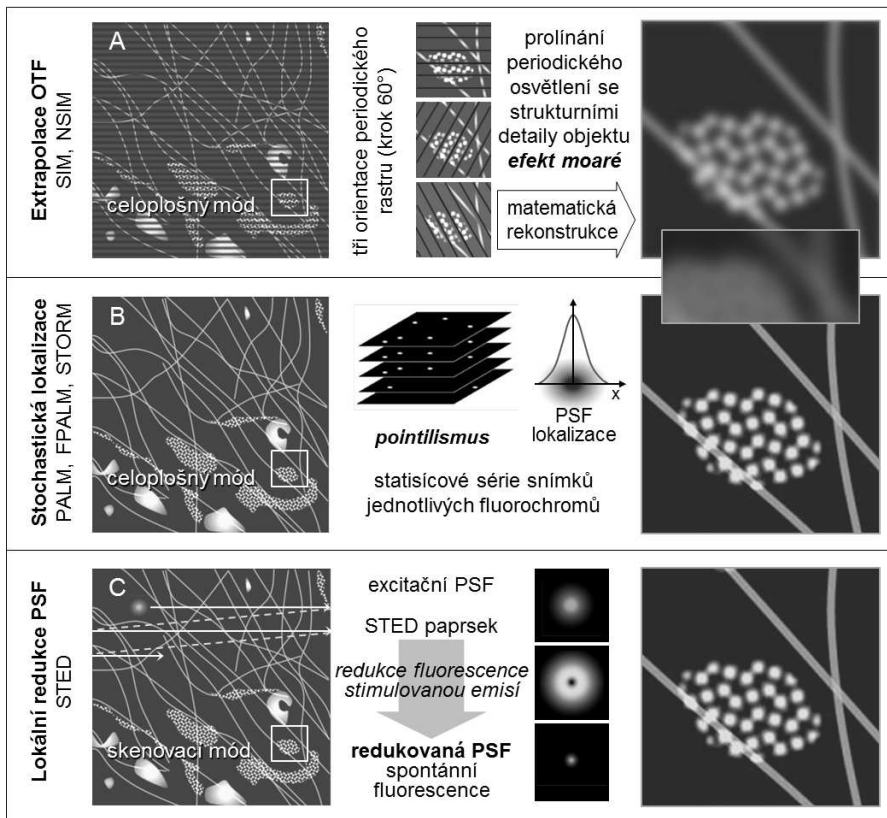
Obr. 4. Tři hlavní strategie superrezoluční mikroskopie: A. celoplošný mód s periodickým strukturálním osvětlením (SIM), B. celoplošný mód se stochastickým zobrazováním individuálních zářících bodů (PALM, FPALM a STORM), C. skenovací mód s redukcí periferní zóny PSF stimulovanou emisí (STED). Ve třech obrázcích levého sloupce je schematicky znázorněna vnitřní struktura hypotetické buňky s mikrotubulárními vlákny a granulárními útvary. Vložené bílé rámečky lokalizují polohu oblasti zobrazené ve zvětšené podobě v pravém sloupci. Vzhled zvětšených obrázků zjednodušeně naznačuje rozdílné možnosti jednotlivých metod. Zatímco obyčejná SIM metoda nabízí pouze dvojnásobné zlepšení rozlišovací schopnosti, které znamená výrazné zlepšení oproti standardní celoplošné mikroskopii (viz vložený segment), ale není ještě dostatečné pro realistické zobrazení rozměrů jemných buněčných struktur, B i C umožňují nanoskopické zobrazení mikrotubulů a dalších struktur o rozměrech blízkých k 20 nm. Volně podle [34].
