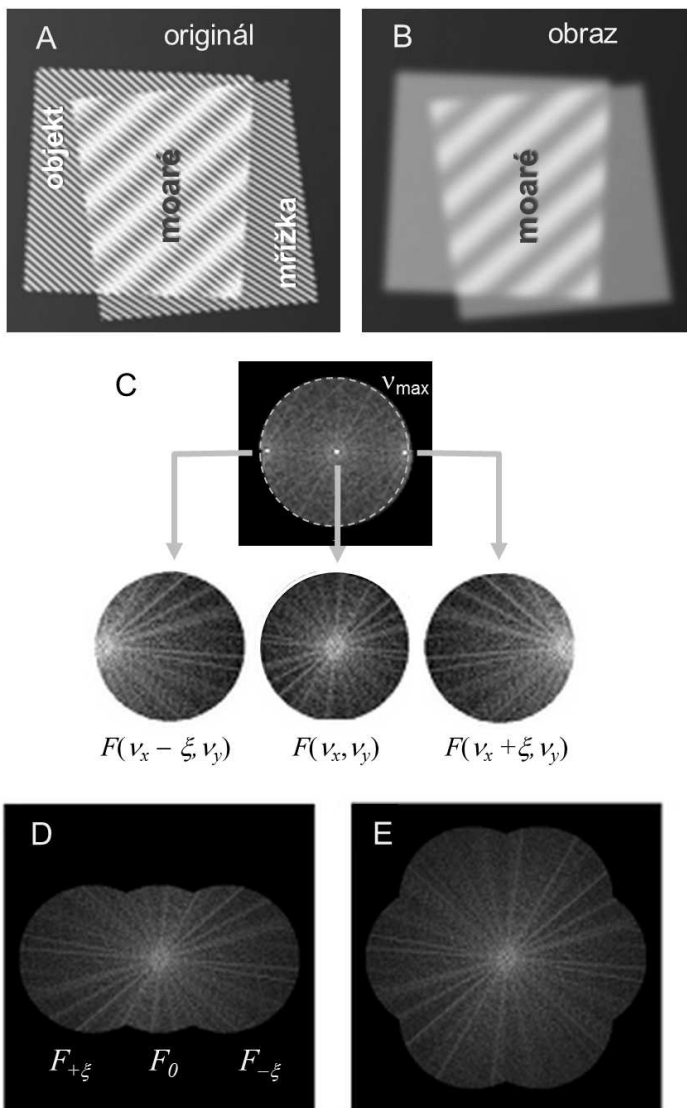
Obr. 5. Princip mikroskopie se strukturálním osvětlením. A. Ukázka moaré efektu vznikajícího překryvem dvou mřížek; B. zobrazení moaré pomocí optické soustavy s rozlišovací schopností menší, než vyžaduje prostorová frekvence mřížek; C. modelový příklad Fourierovy reprezentace objektu osvětleného harmonickou mřížkou o prostorové frekvenci \nu_{\max} a její rozklad na jednu základní a dvě frekvenčně posunuté komponenty (zobrazeny jsou moduly příslušných komplexních funkcí); D. extrapolace Fourierovy transformace F(\nu_x, \nu_y) na rozšířený spektrální interval \langle -2\nu_{\max}, 2\nu_{\max} \rangle ; E. Kombinace extrapolovaných Fourierových transformací získaných pomocí tří orientací osvětlovací mřížky. Vytvořeno s použitím [8].
